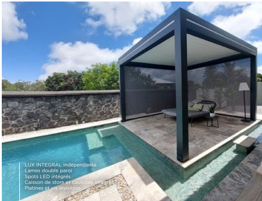
LUX INTEGRAL attenante Lames perpendiculaires double paroi Caisson de store et coulisses intégrés Coulisse murale Platines et vis invisibles
