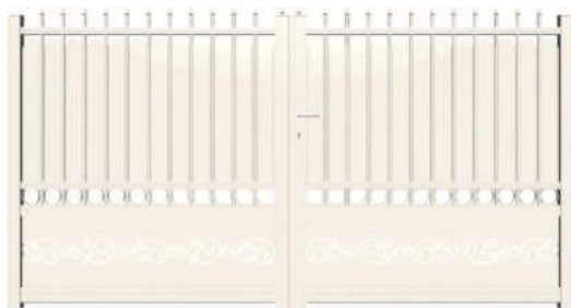
2 vantaux : barreaux Ø 20 mm, tôle ép. 3 mm personnalisée motif Aubade, feston ép. 2 mm et fers de lance pointé Coloris : blanc pur RAL 9010
