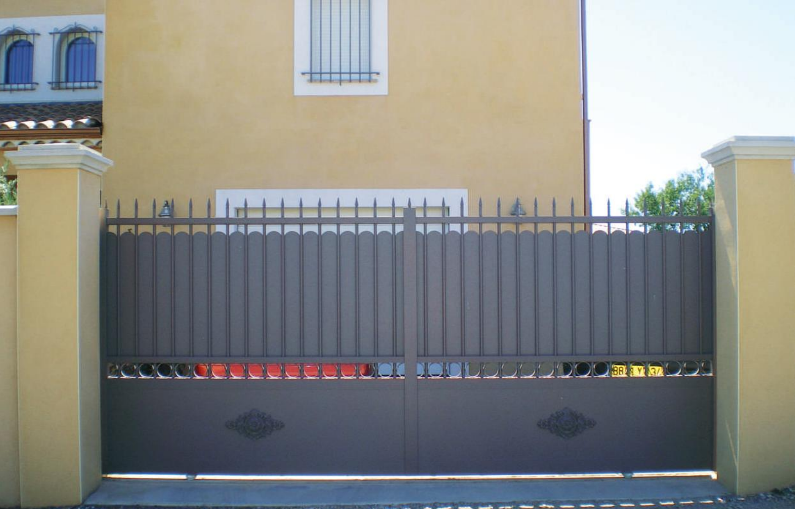
Coulissant Ravel : barreaux Ø 20 mm, tôle ép. 3 mm, feston ép. 2 mm, fers de lance pointés et rosaces Coloris : gris bleu RAL 7031 Finition motorisée
