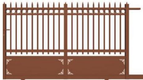
Couissant : barreaux Ø 20 mm, tôle ép. 3 mm personnalisée motifs d'angle Mélodie et fers de lance pointe Coloris : tanami
