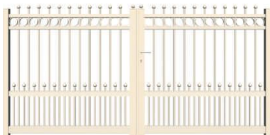
2 vantaux : barreaux Ø 20 mm et fers de lance goutte d'eau Coloris : ivoire clair RAL 1015
