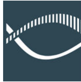
ADN (5)
